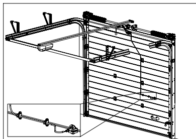
Рис. 6. Механизм разблокировки
