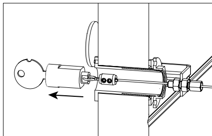
Рис. 6. Механизм разблокировки
