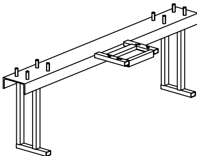
Рис. 3. Рама ворот опорная FLGU.400.0826
