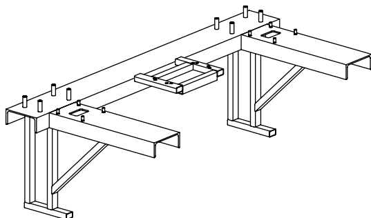
Рис. 1. Рама ворот опорная FLGU.400.0821
