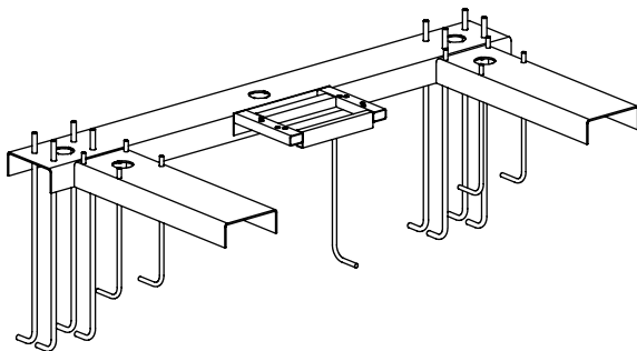
Рис. 5. Рама ворот опорная FLGU.400.0824
