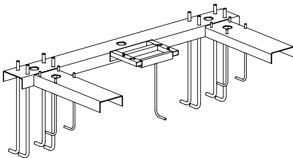
Рис. 2. Рама ворот опорная FLGU.400.0823
