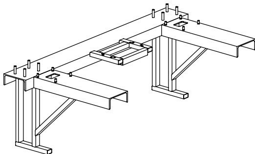
Рис. 4. Рама ворот опорная FLGU.400.0822
