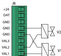
Рисунок 6. Подключение клапанов
