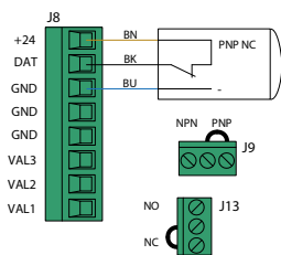
Рисунок 8. Подключение датчика положения ворот:
