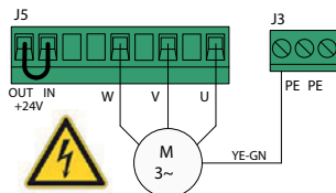
Рисунок 5. Подключение электродвигателя
