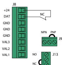
Рисунок 8. Подключение датчика положения ворот:
