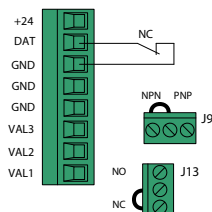
Рисунок 7. Подключение кнопок управления и светодиода (рис. 1)
