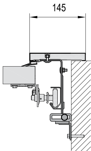
Монтаж перед проемом Комплект арт. FWO145/145-40
