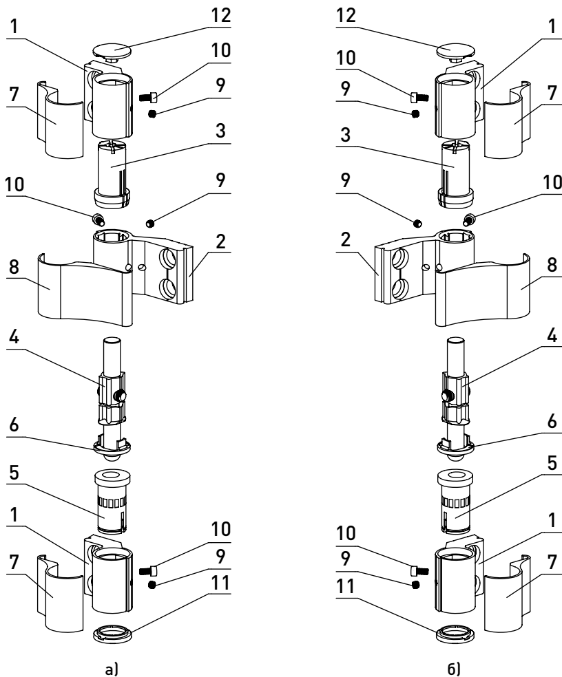
Рис. VII. Сборка петли ЗАH67 :
