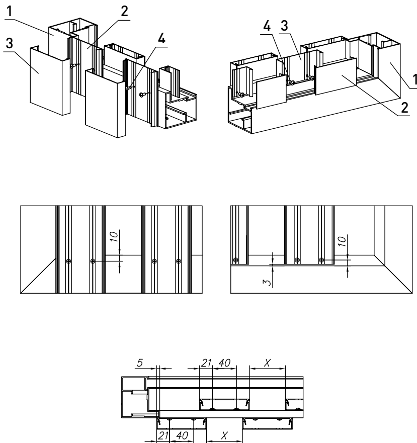
Рис. 29а. Шахматное заполнение профилями шириной 82 мм
