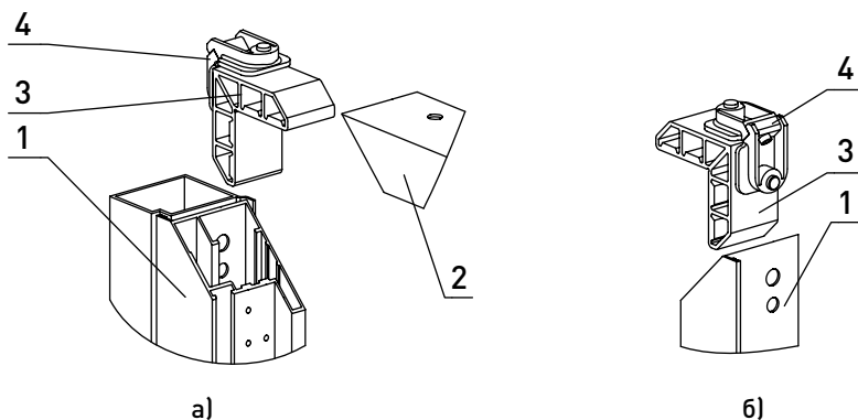
Рис. 7. Установка соединителей:
