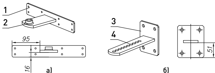
Рис. 62. Изготовление кронштейнов для установки электроприводов:
