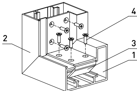
Рис. 11. Крепление углов
