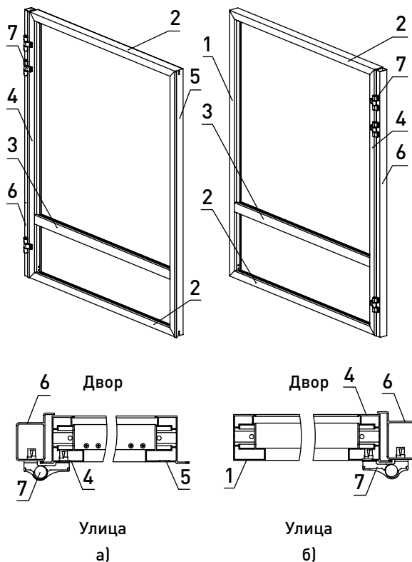
Рис. 3. Рамы распашных ворот с видом открывания наружу:
