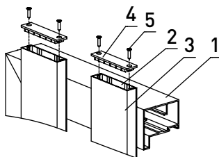
Рис. 34. Установка крышек FLGU.400.0702
