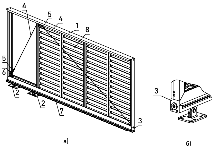
Рис. 11. Створка ворот:
