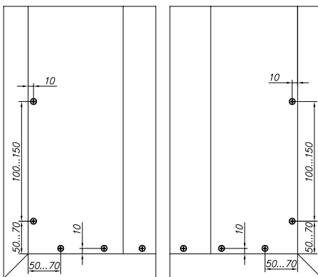
Рис. 15.2. Схема разметки вертикально установленных панелей
