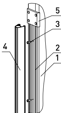
Рис. 44. Установка демпфирующего элемента:
