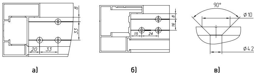
Рис. 9. Изготовление отверстий:
