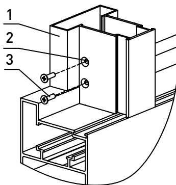
Рис. 8. Крепление импоста:
