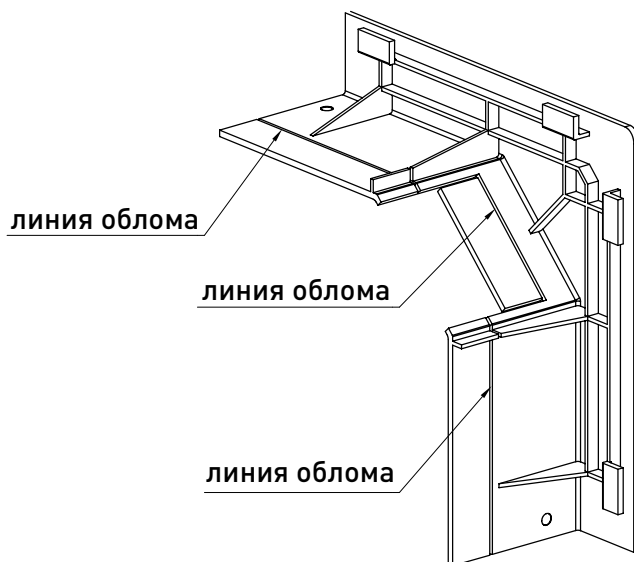
Рис. 21. Крышка FLGU.400.0717
