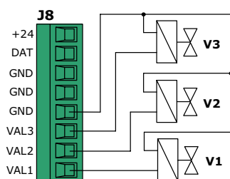
Рисунок 6. Подключение клапанов
